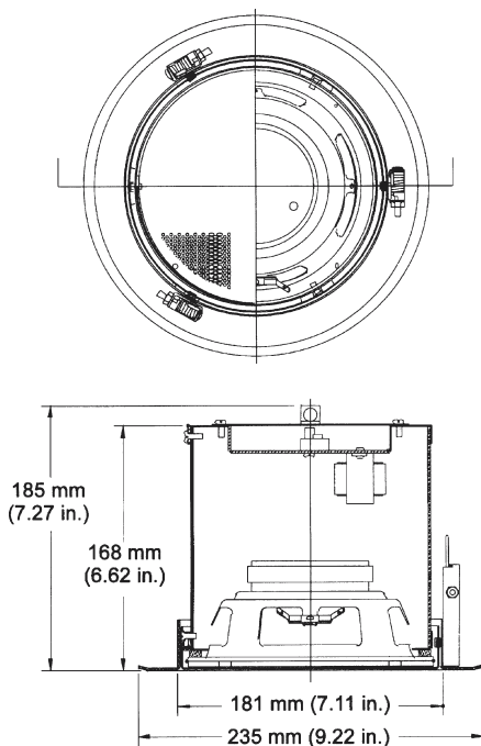
Dimensions
