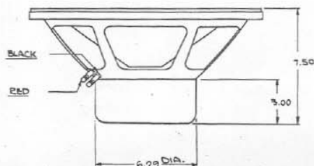
Fig. 1 — Dimensions
