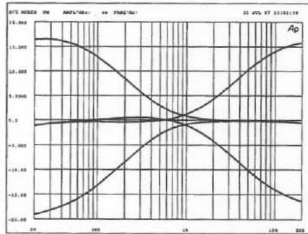
LOW-HI EQ
