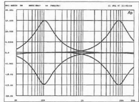
MID EQ
