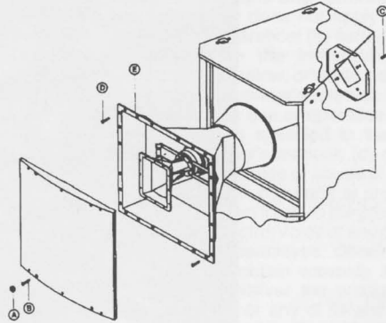
FIGURE 5 — Module Rotation
