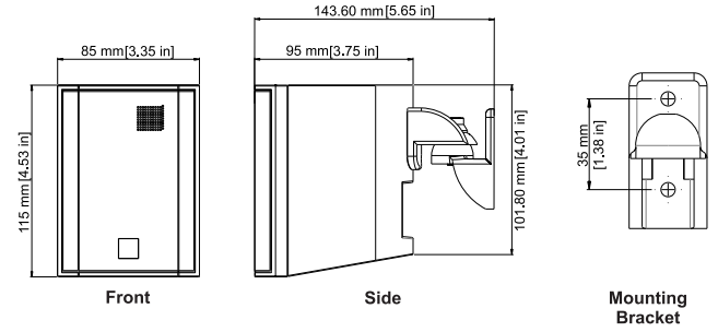
EVID-2.1-järjestelmän ja kiinnikkeen mitat
