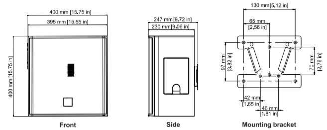
EVID-40S-järjestelmän ja kiinnikkeen mitat
