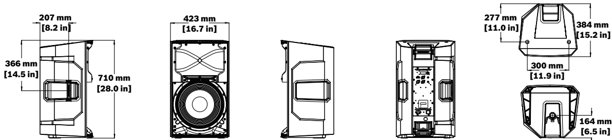
图片 9.3: ELX200-15P 尺寸
