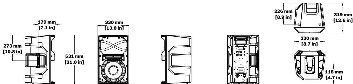
图片 9.1: ELX200-10P 尺寸
