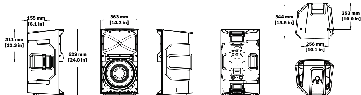
图片 9.2: ELX200-12P 尺寸
