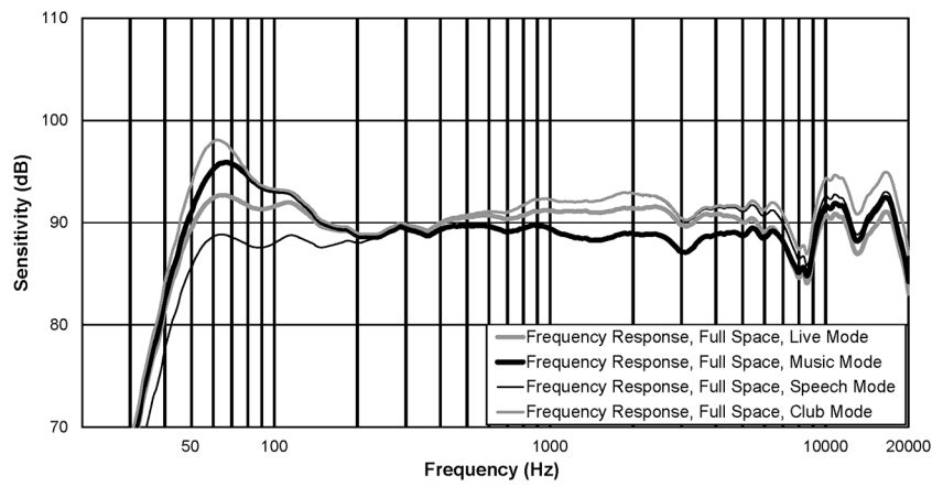
Abbildung 9.3: Frequenzgang EVOLVE 50 (Live, Music, Speech und Club)
