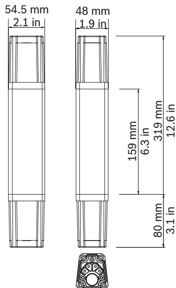
Abbildung 9.2: Abmessungen EVOLVE 50 kurzer Mast
