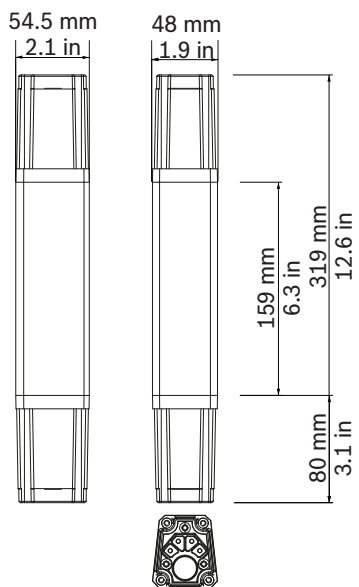
图片 9.2: EVOLVE 50短支撑杆的尺寸
