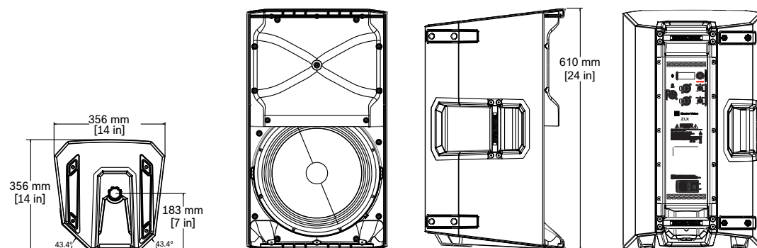
Abbildung 7.1: Abmessungen ZLX-12BT
