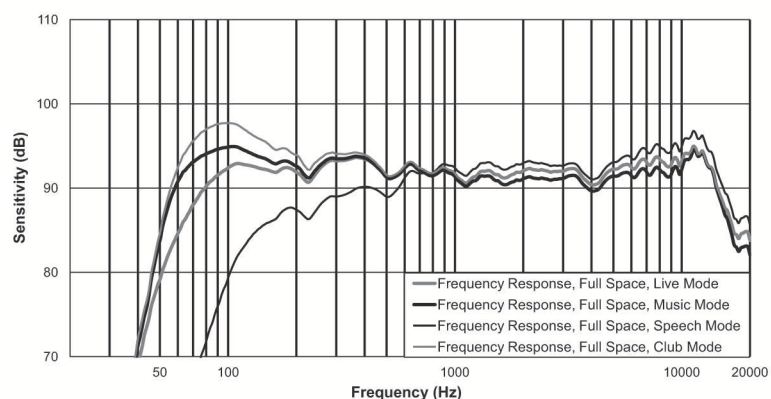
Abbildung 7.3: Frequenzgang ZLX-12BT
