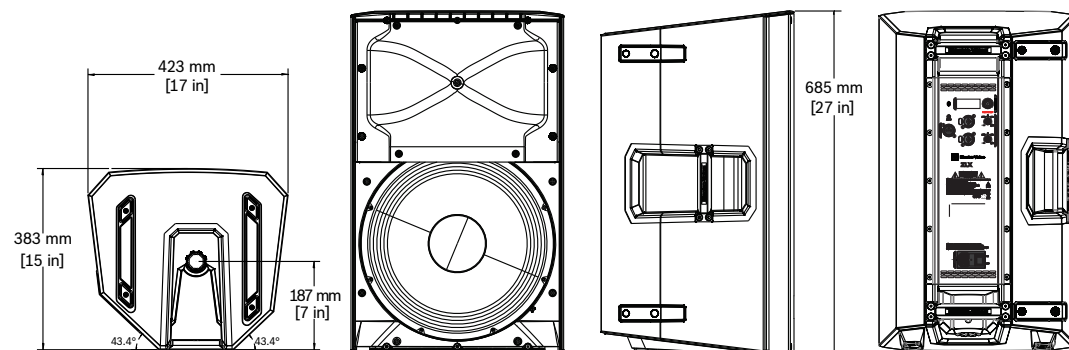
Abbildung 7.2: Abmessungen ZLX-15BT
