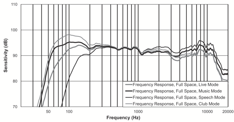
Abbildung 7.4: Frequenzgang ZLX-15BT
