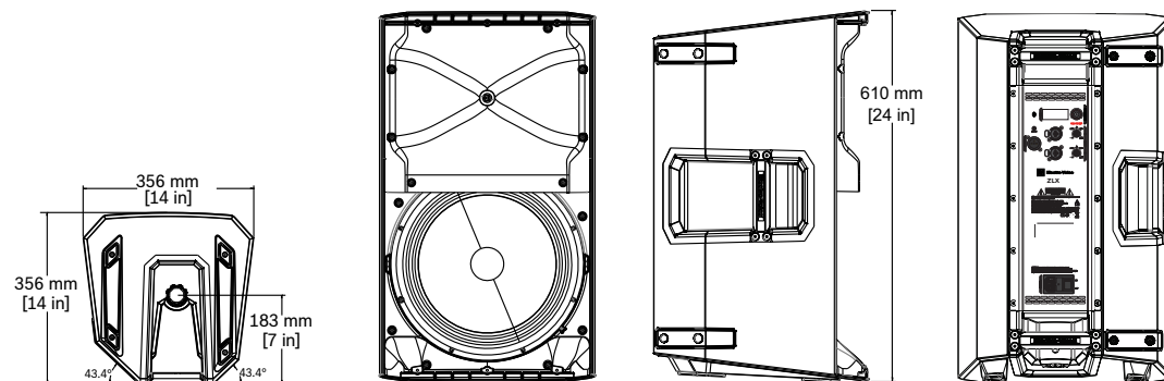
Figura 7.1: Dimensiones ZLX-12BT
