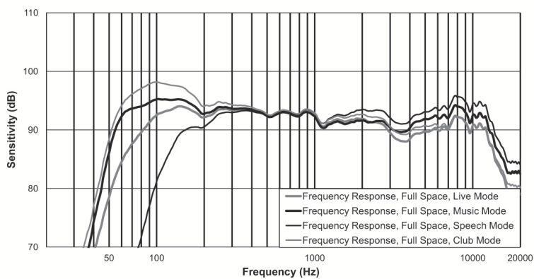
Figura 7.4: Respuesta de frecuencia ZLX-15BT
