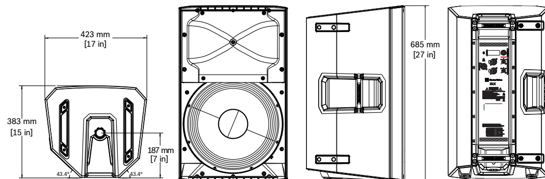
Figura 7.2: Dimensiones ZLX-15BT
