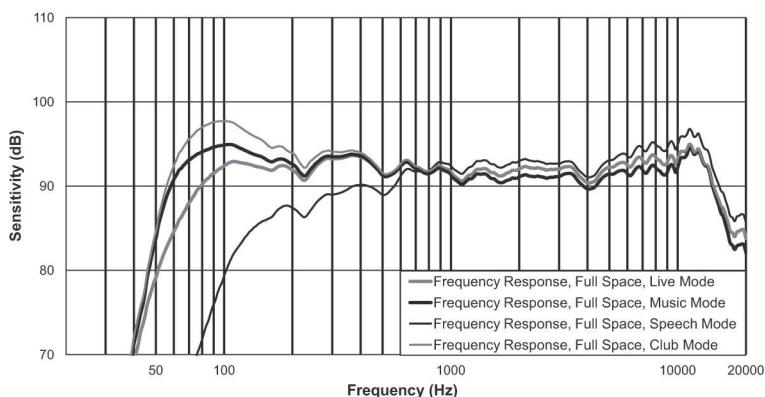
Figura 7.3: Respuesta de frecuencia ZLX-12BT
