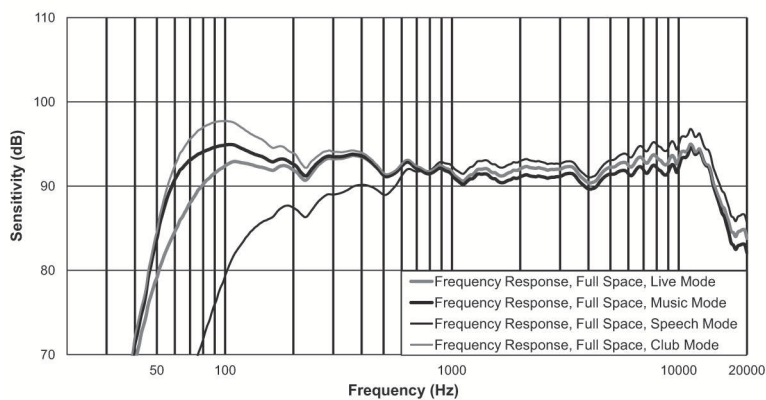
図 7.3: 周波数特性 ZLX-12BT
