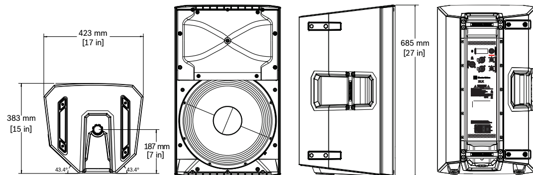
図 7.2: 寸法 ZLX-15BT
