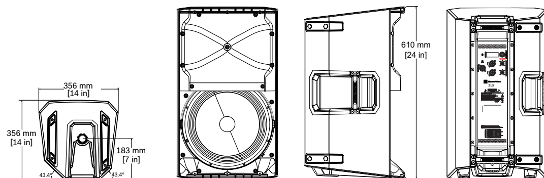
図 7.1: 寸法 ZLX-12BT
