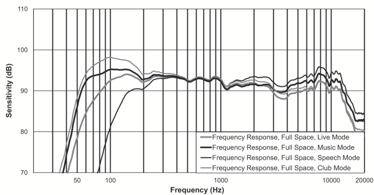
図 7.4: 周波数特性 ZLX-15BT
