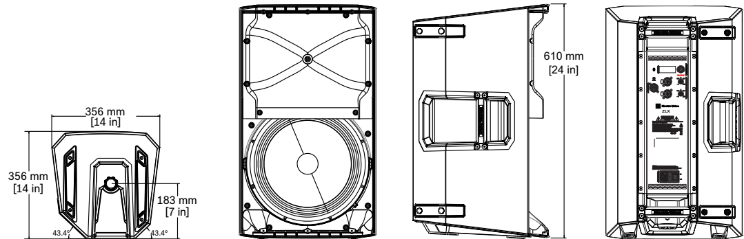
그림 7.1: 치수 ZLX-12BT
