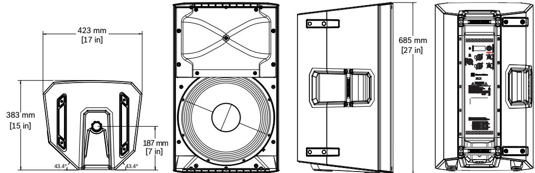
그림 7.2: 치수 ZLX-15BT
