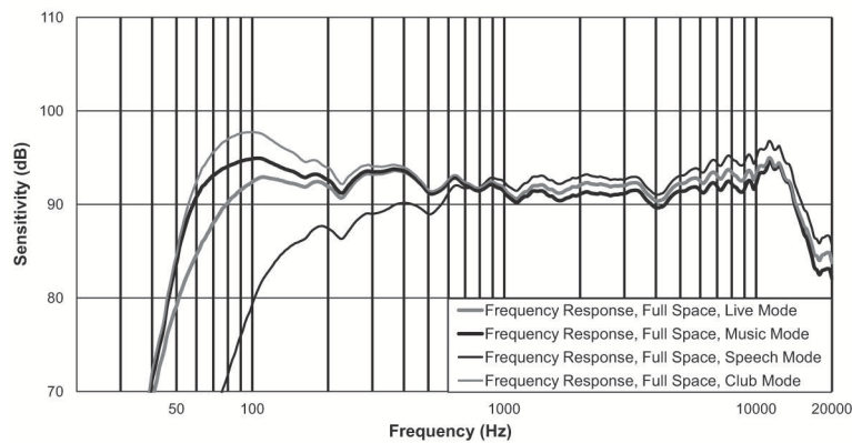
그림 7.3: 주파수 응답 ZLX-12BT
