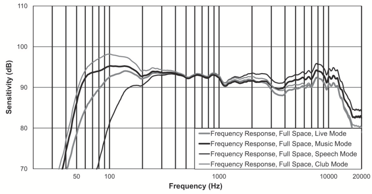
그림 7.4: 주파수 응답 ZLX-15BT
