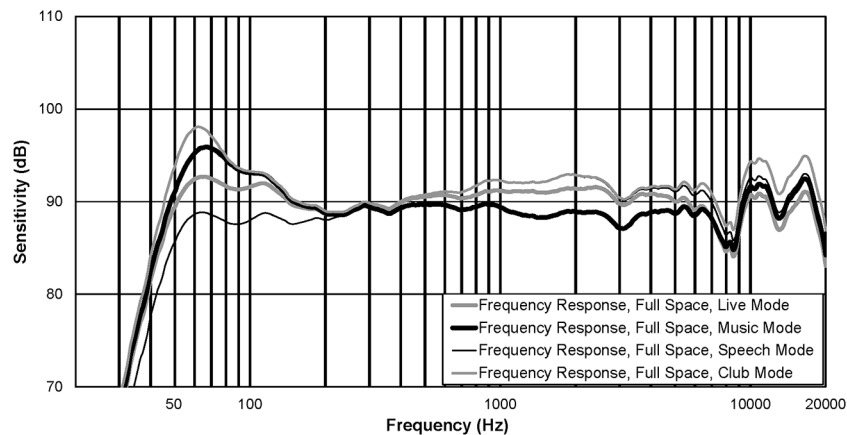
図 10.1: 周波数特性 EVOLVE 50M (Live モード、Music モード、Speech モード、Club モード)
