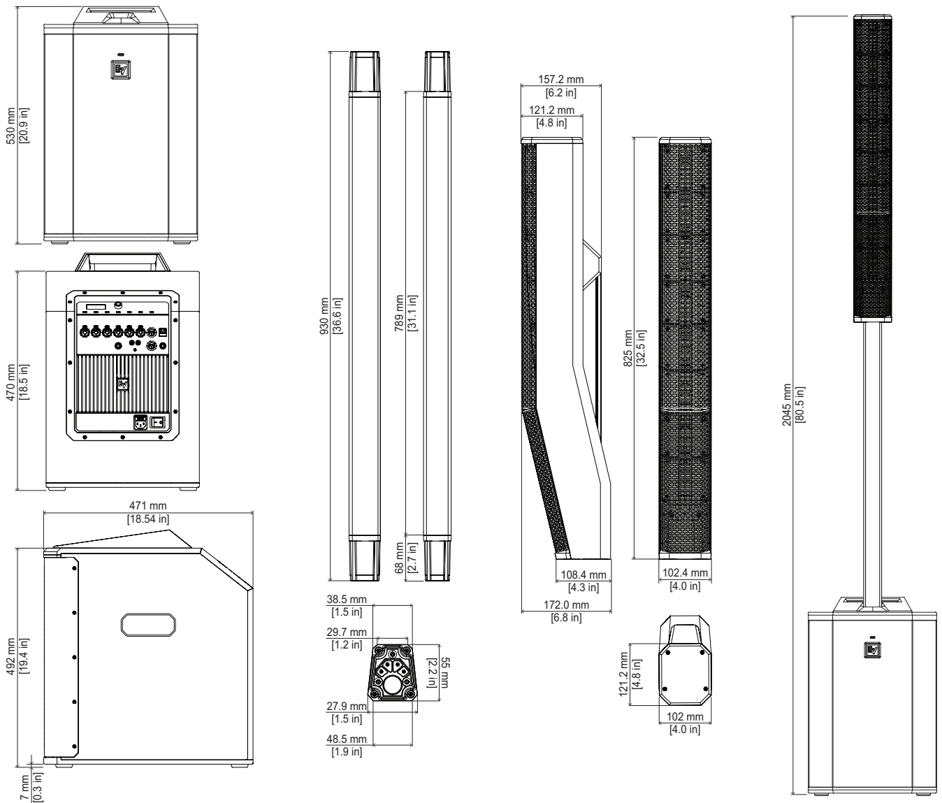
図 10.2: 寸法 EVOLVE50M システム
