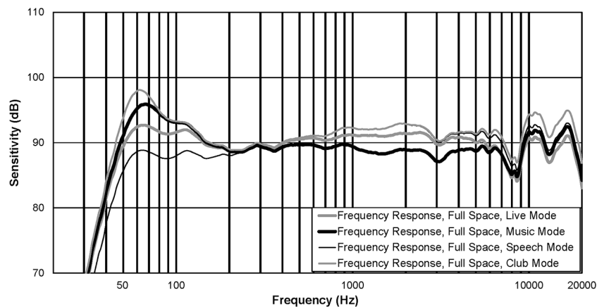
图片 10.1: 频率响应EVOLVE 50M (“Live” (现场)、“Music” (音乐)、“Speech” (人声)和“Club” (俱乐部)模式)
