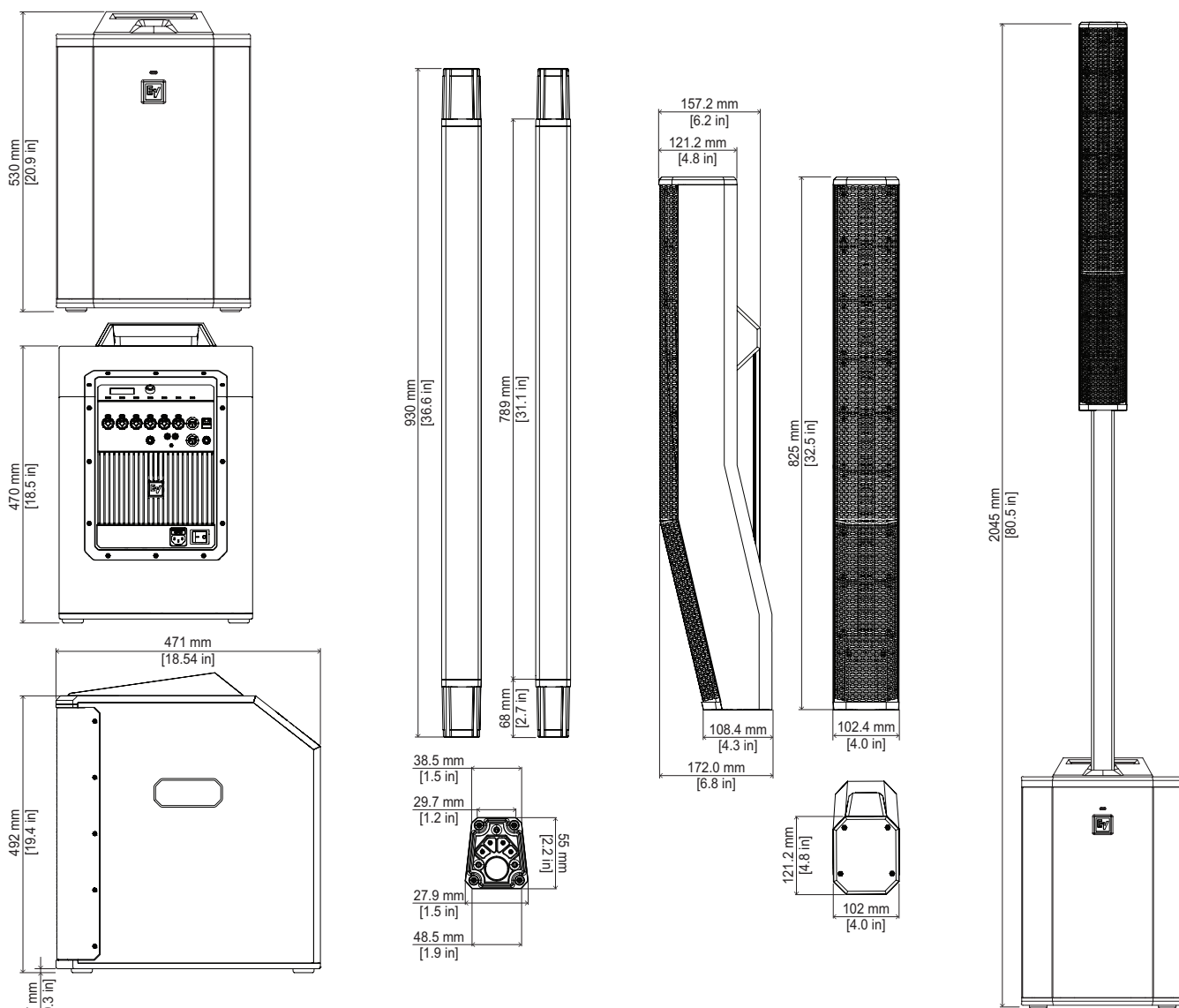
图片 10.2: EVOLVE50M系统尺寸
