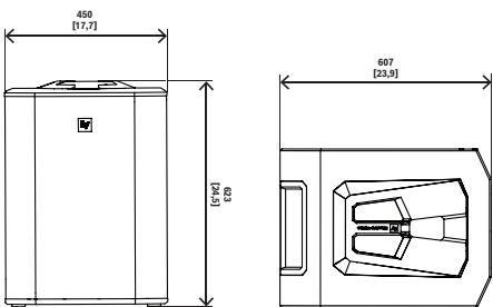
Fig. 3: Poste EVOLVE70-90
