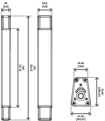
Fig. 3: Poste EVOLVE70-90
