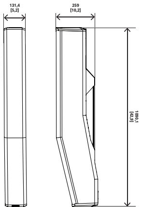
Fig. 2: Columna EVOLVE70-90
