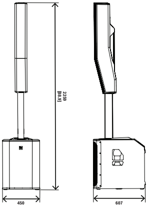
Fig. 1: Sistema EVOLVE 70
