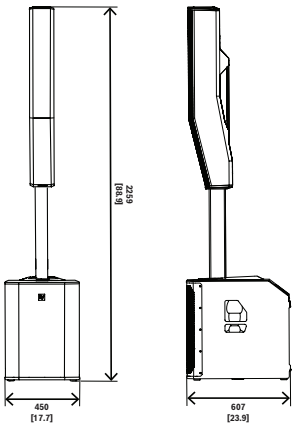
図 1: EVOLVE 70 システム
