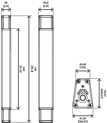
図 3: EVOLVE70-90 ポール
