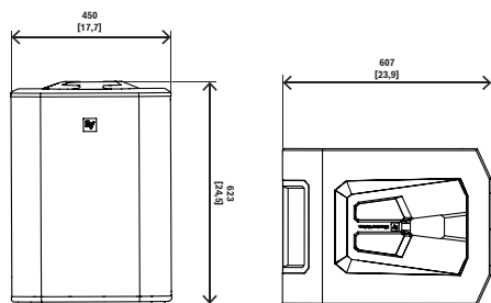
図 4: EVOLVE 70 サブウーファー
