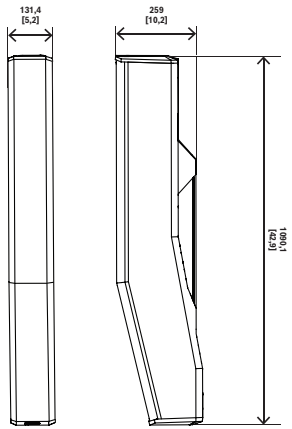
図 2: EVOLVE70-90 カラム
