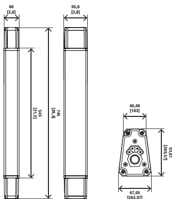
3: EVOLVE70-90 폴
