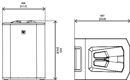
4: EVOLVE 70 서브우퍼
