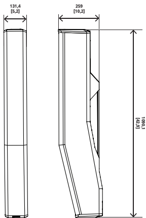
2: EVOLVE70-90 칼럼
