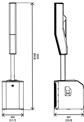
1: EVOLVE 70 시스템
