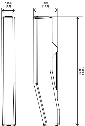
图 2: EVOLVE70-90 音柱
