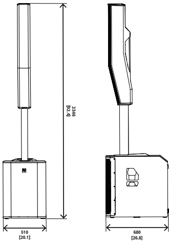
图 1: EVOLVE 90 系统
