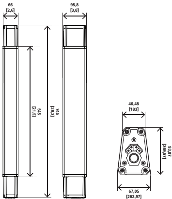
图 3: EVOLVE70-90 立杆
