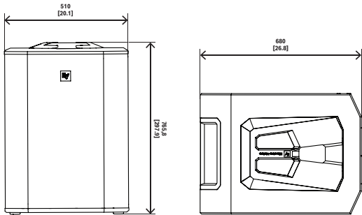
图 4: EVOLVE 90 低音炮
