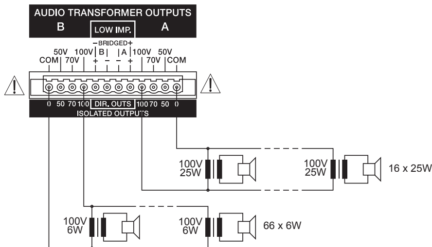
Beispielbeschriftung PA2400T mit 100V Lautsprechern. Maximale Auslastung mit Lautsprechern 25W/100V und 6W/100V.
