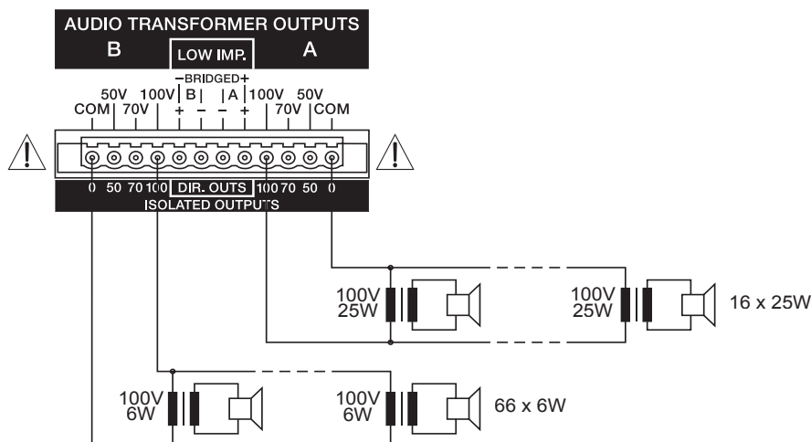
Exemple de configuration : PA2400T avec haut-parleur de 100V connecté. Charges de travail maximum avec haut-parleurs de 25W/100V et 6W/100V.
