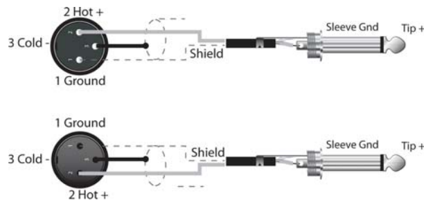
Abbildung 3-2: Unsymmetrisches XLR auf Klinke Kabel
