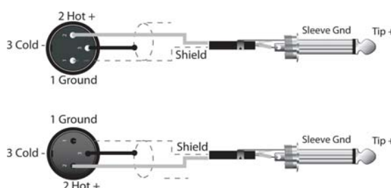
Illustration 3-2: Câbles audio non symétrisés
