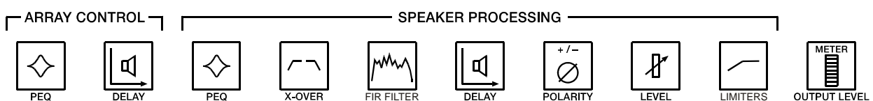
Abbildung 5-6: DSP-Blöcke in Ausgang 1 bis 6
