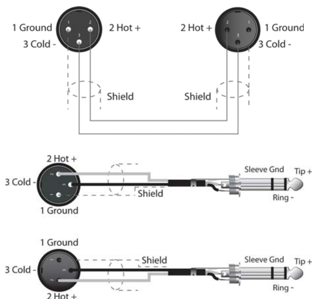
Abbildung 3-1: Symmetrisches XLR auf XLR Kabel bzw. XLR auf Klinke Kabel
