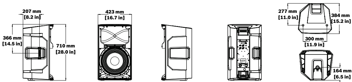
図 9.3: ELX200-15P の寸法
