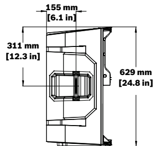
그림 9.2: ELX200-12P 크기
