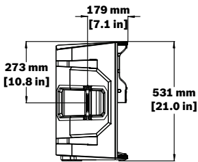
그림 9.1: ELX200-10P 크기
