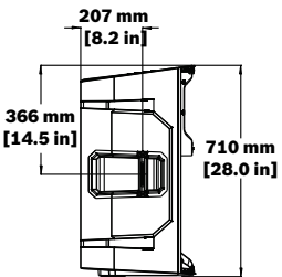
그림 9.3: ELX200-15P 크기
