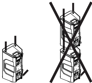
그림 4.5: 스피커 수직 서스펜션(왼쪽은 맞고, 오른쪽은 잘못됨)
