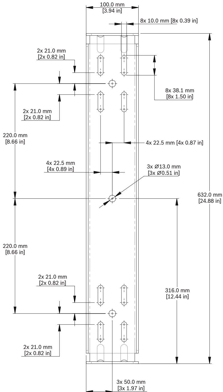
Abbildung 5.1: Abmessungen – 10"-U-Halterung
