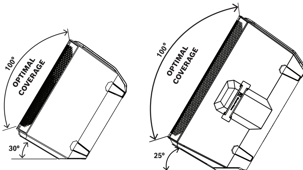
Abbildung 4.3: EVERSE 8 und optimale EVERSE 12-Abdeckung in der Kickback-Position
