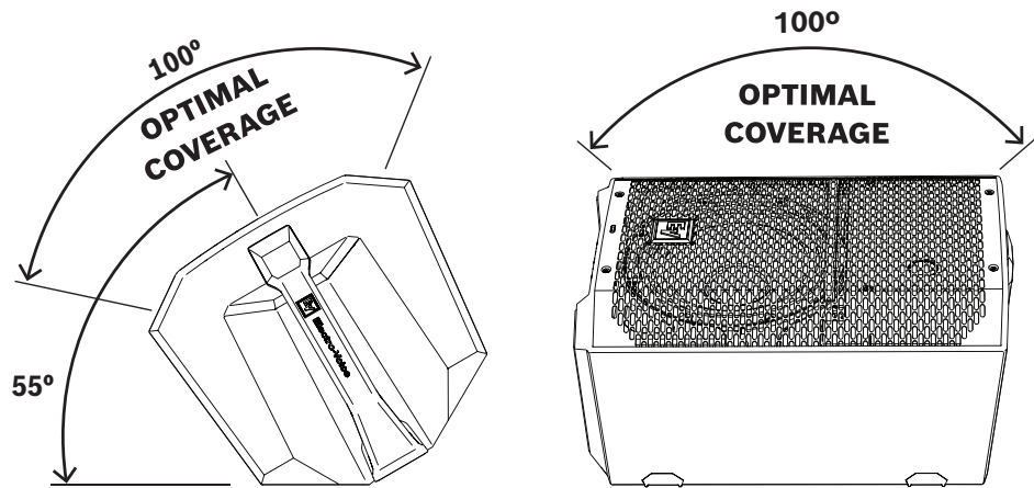
Figure 4.1: EVERSE 8 - Couverture optimale en retour de scène (vue latérale gauche et vue avant droite)
