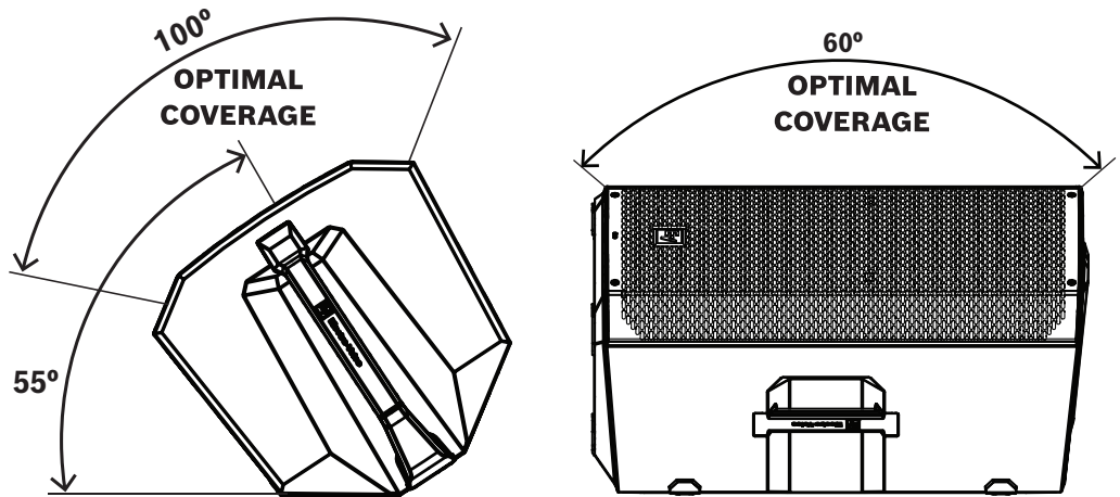
Figure 4.1: EVERSE 8 - Couverture optimale en retour de scène (vue latérale gauche et vue avant droite)
